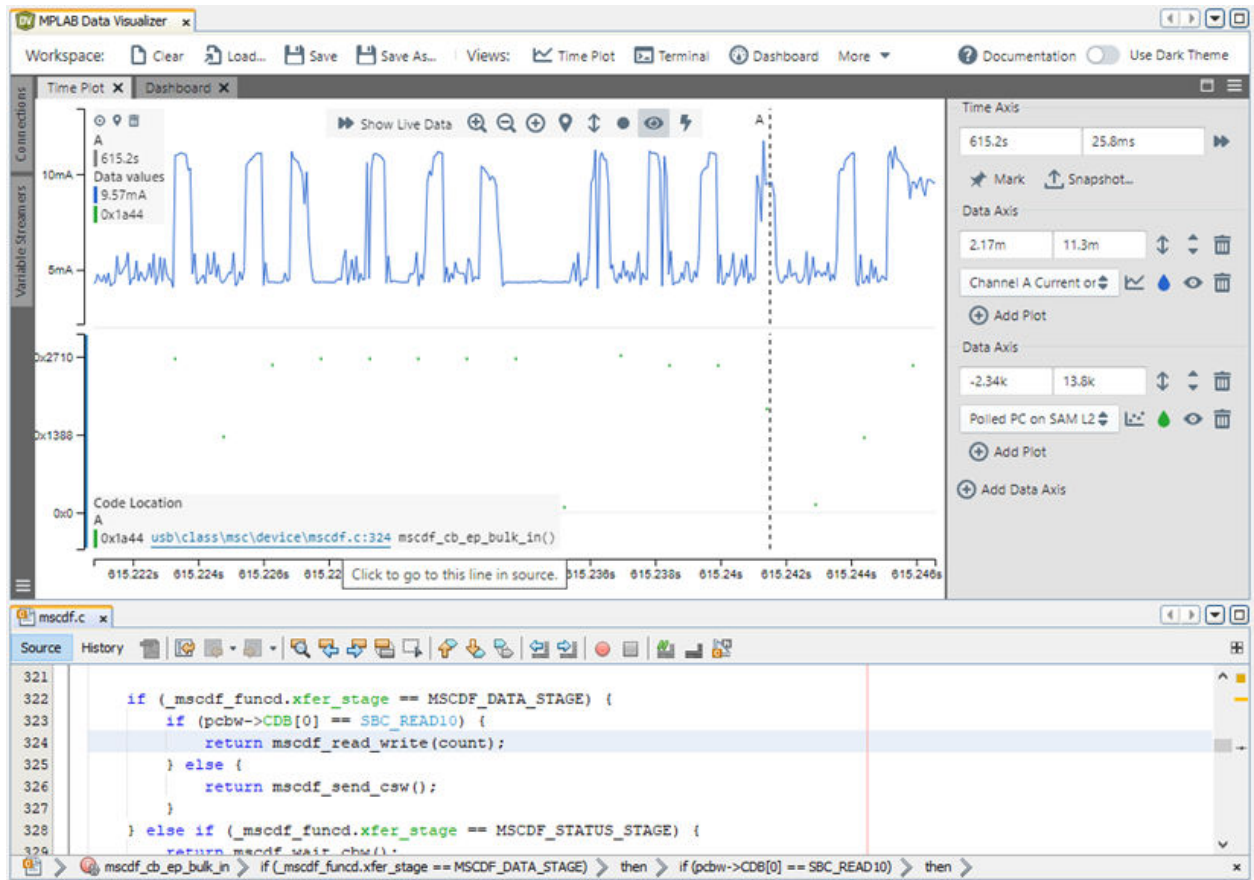
图 4-35. PC 值和源代码位置
