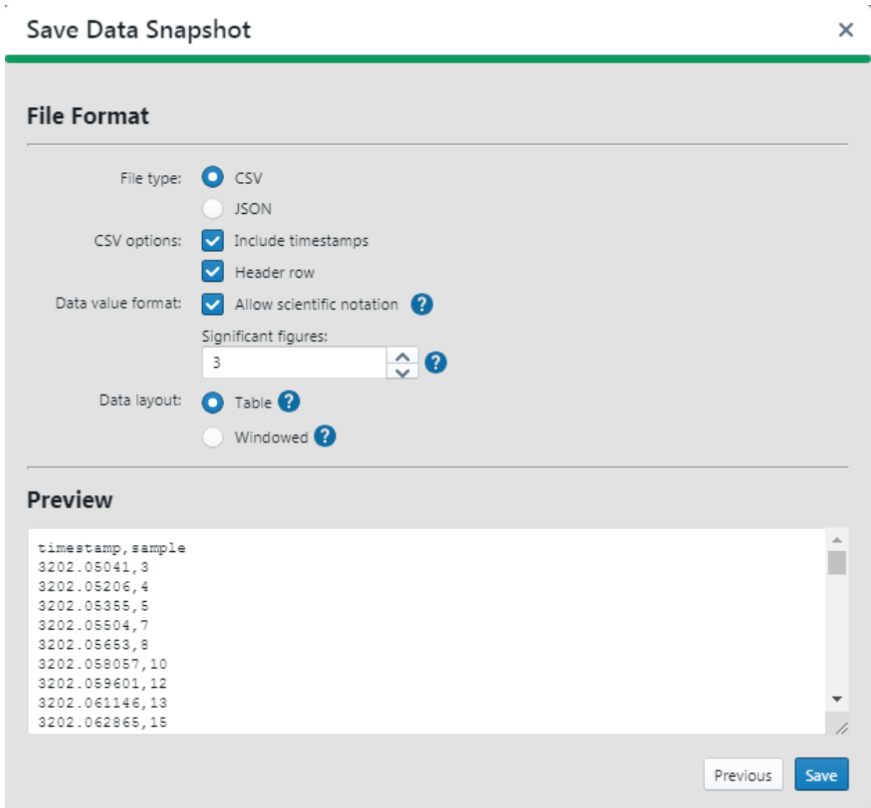
图 4-21. Snapshot——File Format（文件格式）
