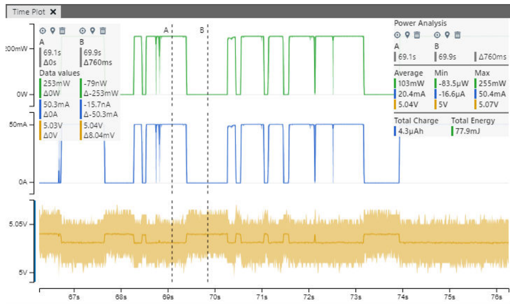
图 4-29. 使用功率分析的值
