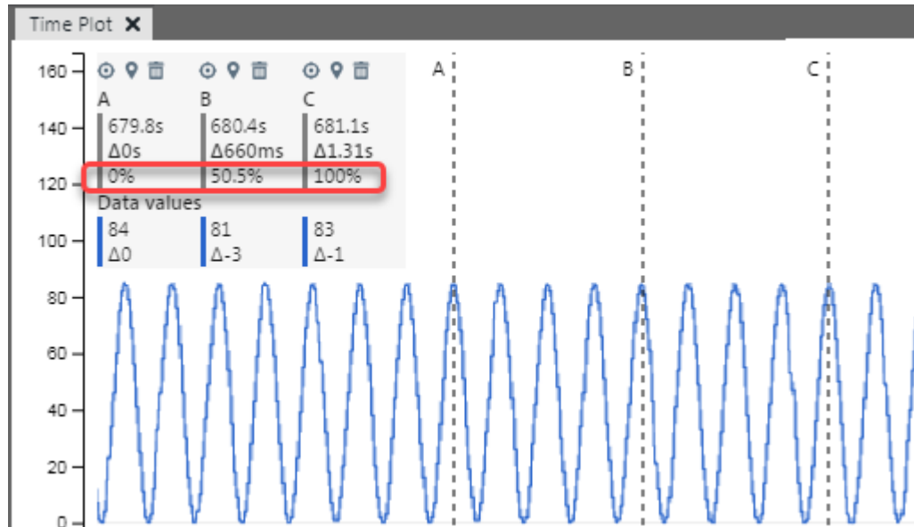
图 4-11. 添加三个垂直光标——占空比
