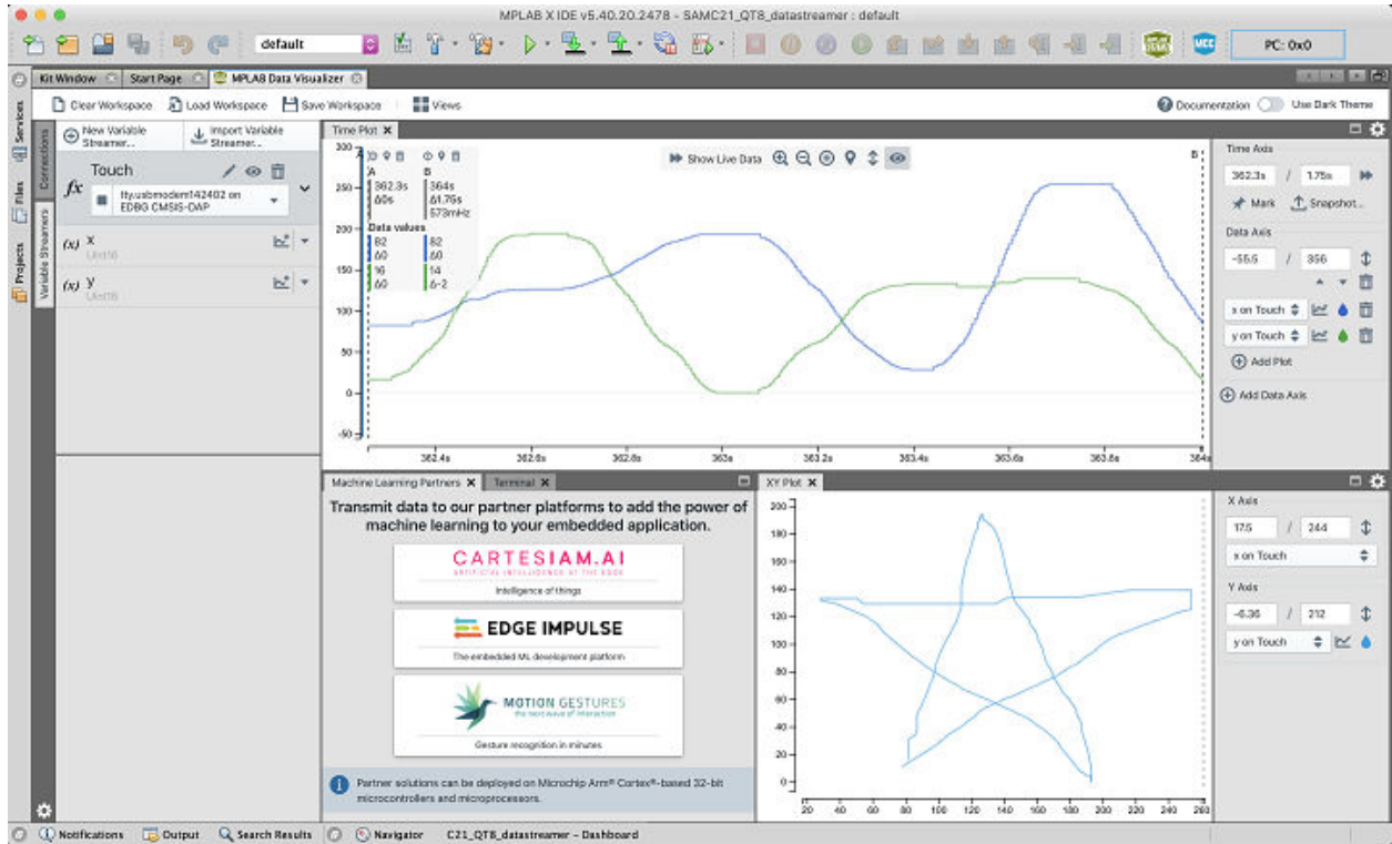
图 4-38. 机器学习插件
