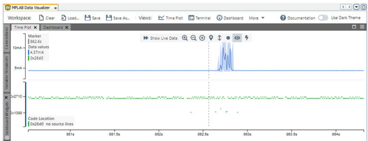
图 4-34. PC 采样和功率性能分析
