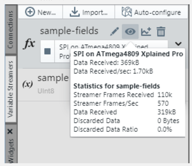
图 4-16. 查看解码统计信息
