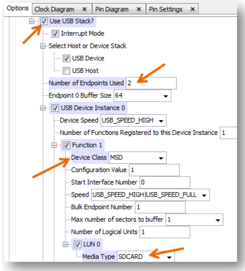
图 2-2. USB 协议栈配置
